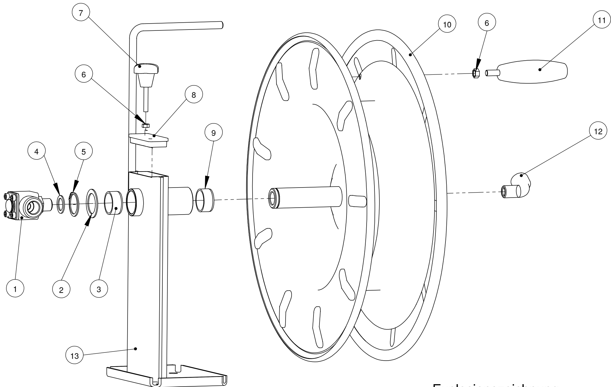
Explosionszeichnung Schlauchaufroller Type STK
